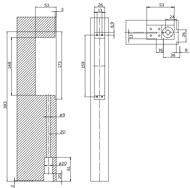
Рисунок 2 Пассивная створка
