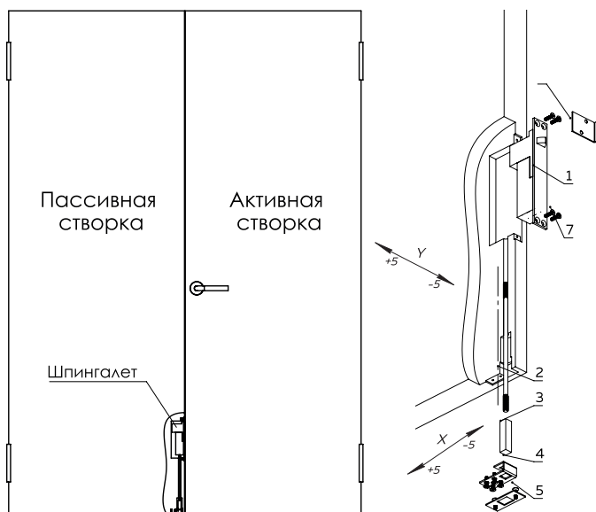
Рисунок 1 – Шпингалет
