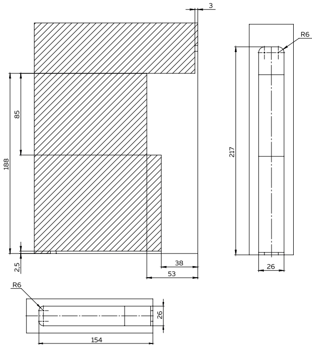
Рисунок 2 Пассивная створка
