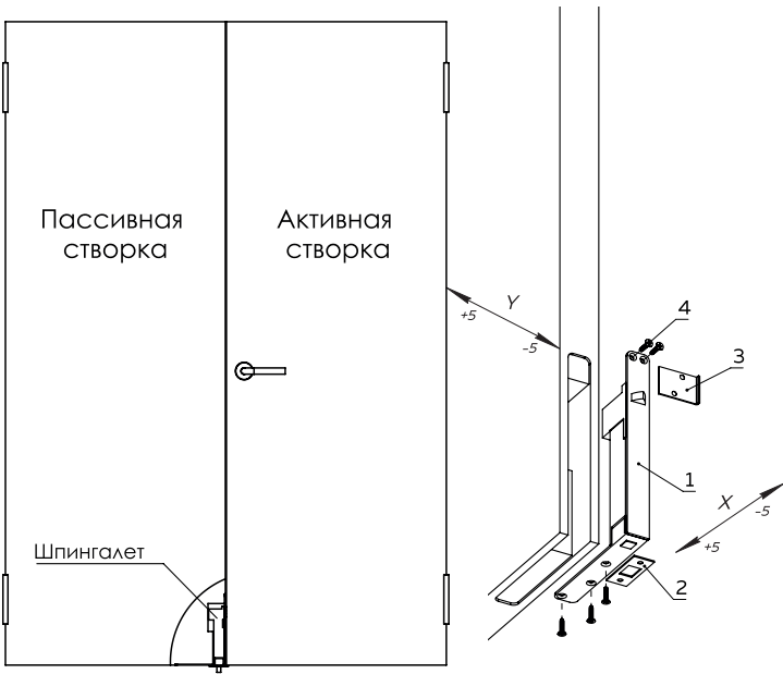
Рисунок 1 – Шпингалет
